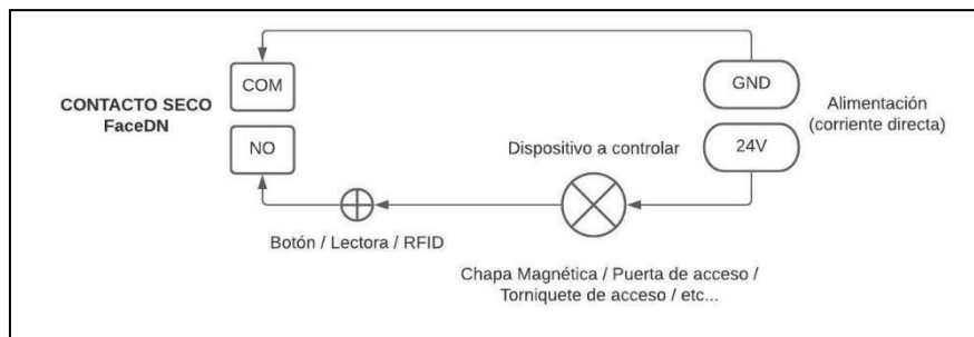
Ilustración 8: Diagrama de conexión contacto seco FaceDN-02 en serie con interruptor adicional de control.
