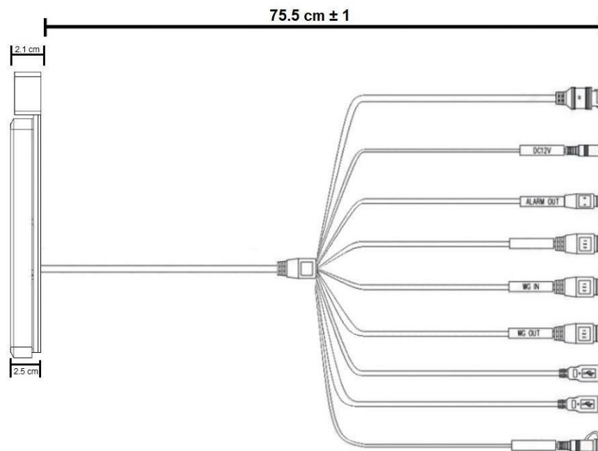
Ilustración 2: FaceDN-02 Pared Vista Lateral.
