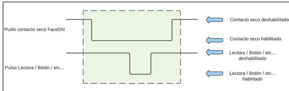
Ilustración 9: Pulso de FaceDN-02 dentro del mismo intervalo de tiempo que el pulso del dispositivo interruptor adicional.
