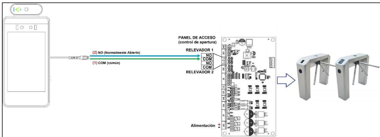
Ilustración 12: Diagrama de referencia para uso de contacto seco de FaceDN-02 utilizando un sistema central de control de acceso.
