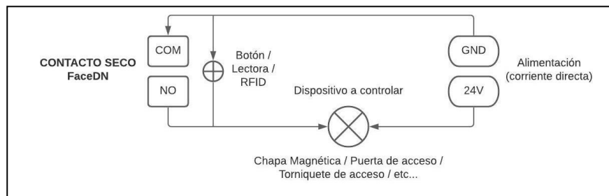
Ilustración 11: Diagrama de conexión contacto seco en paralelo a interruptor adicional de control.
