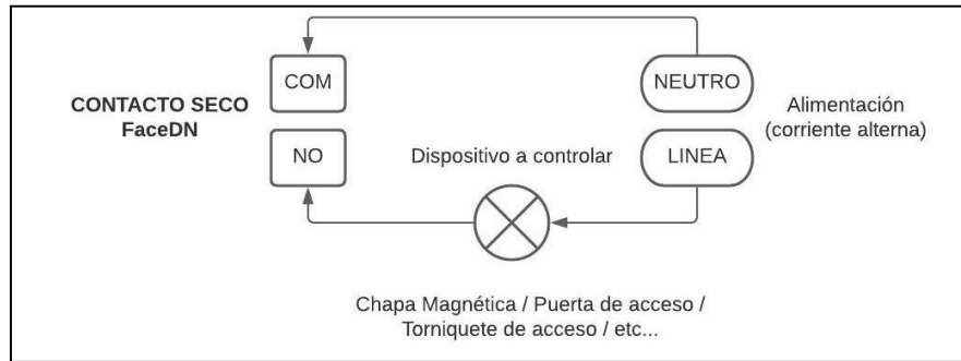
Ilustración 7: Diagrama de conexión serie para uso de contacto seco de FaceDN-02 con alimentación AC.
