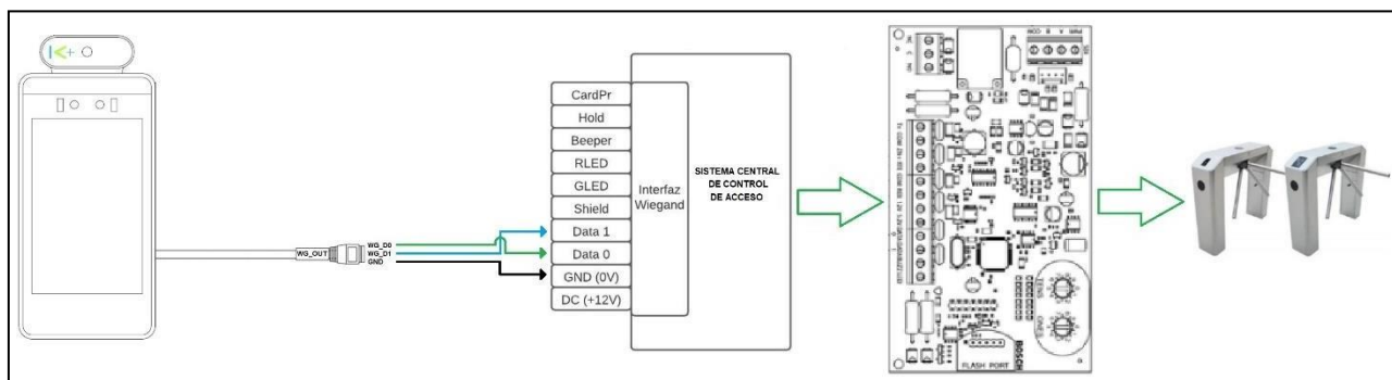
Ilustración 15: Diagrama de referencia para uso de Wiegand en FADN-02 utilizando un sistema central de control de acceso.
