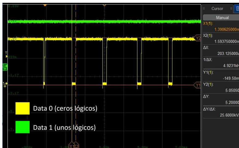
Ilustración 13: Duración de un bit (pulso) de una trama Wiegand al hacer un reconocimiento facial con éxito en FaceDN-02.
