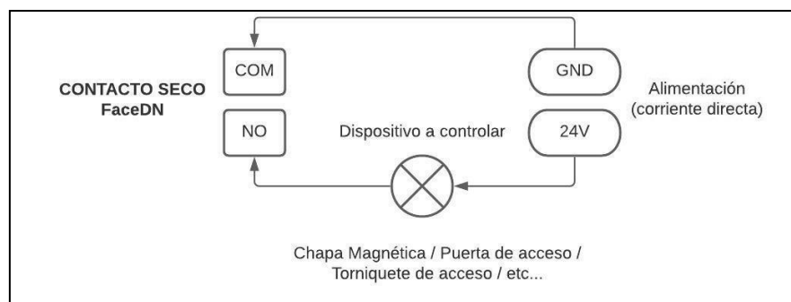
Ilustración 6: Diagrama de conexión serie para uso de contacto seco de FaceDN-02 con alimentación DC.
