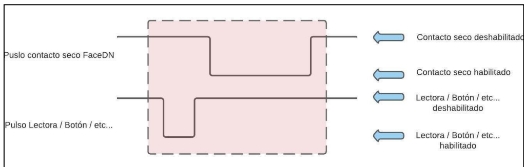
Ilustración 10: Pulso de FaceDN-02 y pulso de dispositivo interruptor de control adicional NO están dentro del mismo intervalo de tiempo.
