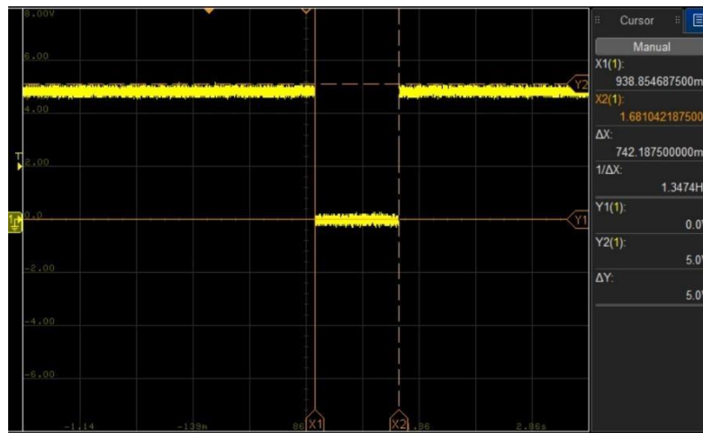
Ilustración 5: Señal del contacto seco al hacer reconocimiento facial con éxito.
